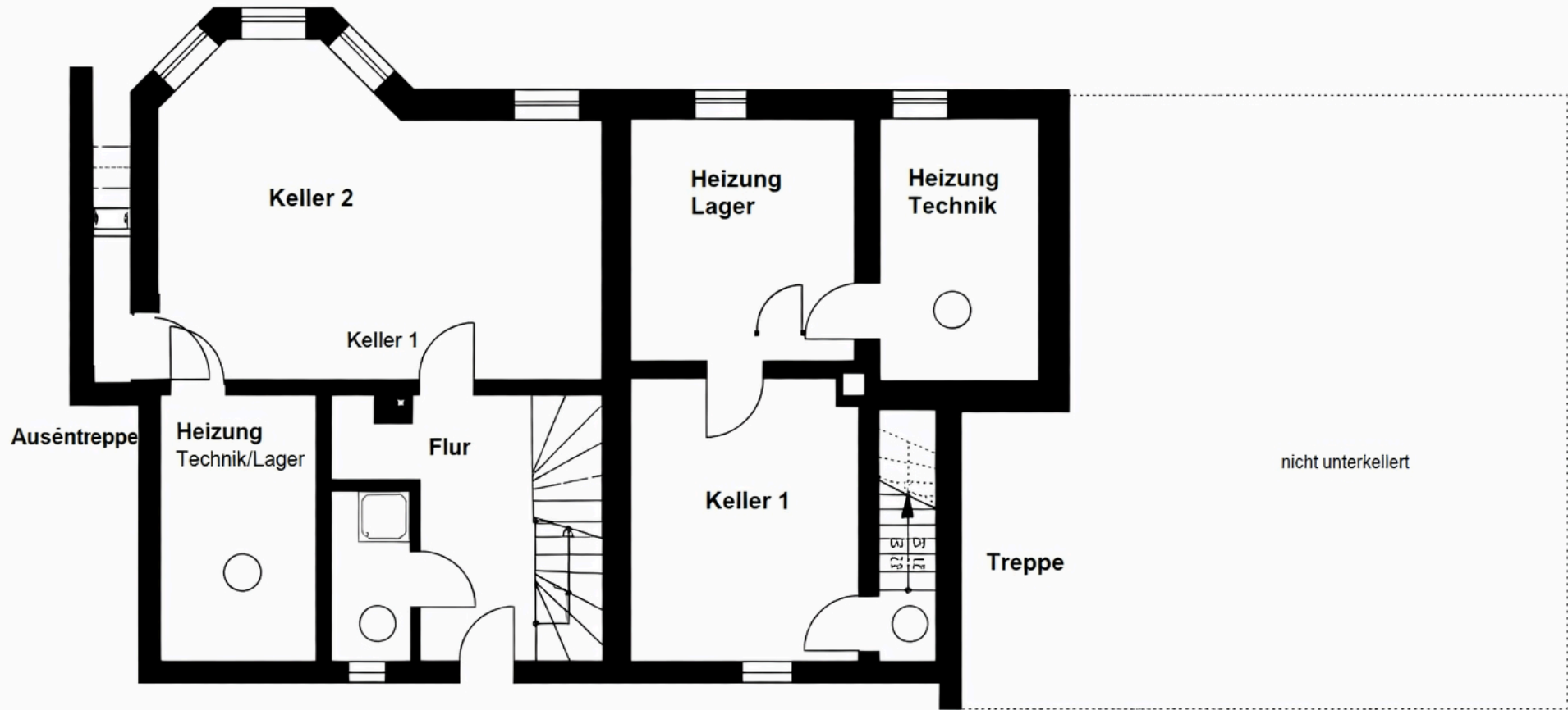
Kellergeschoss
