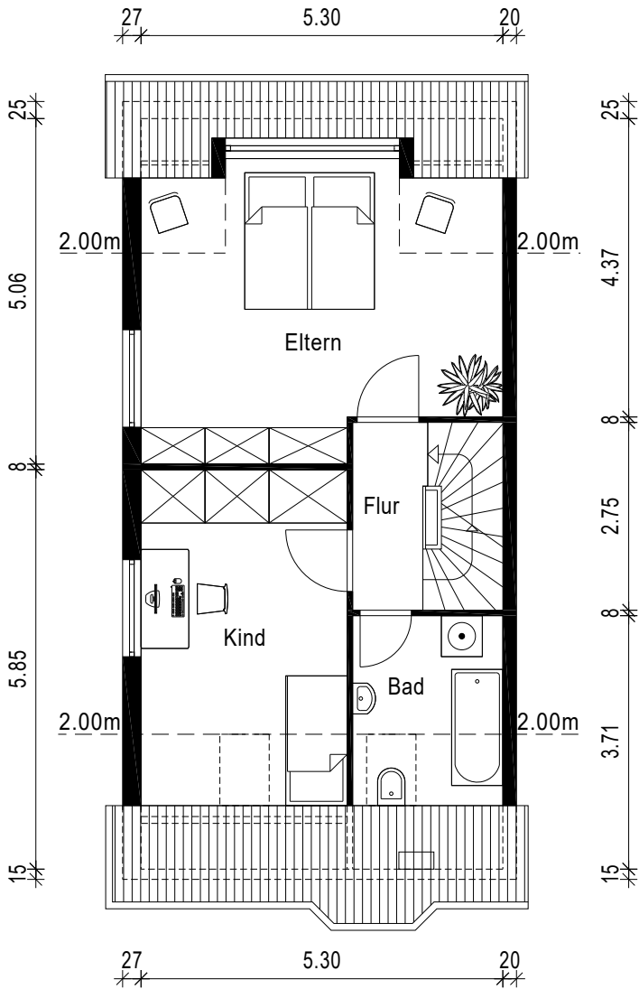
Dachgeschoss
