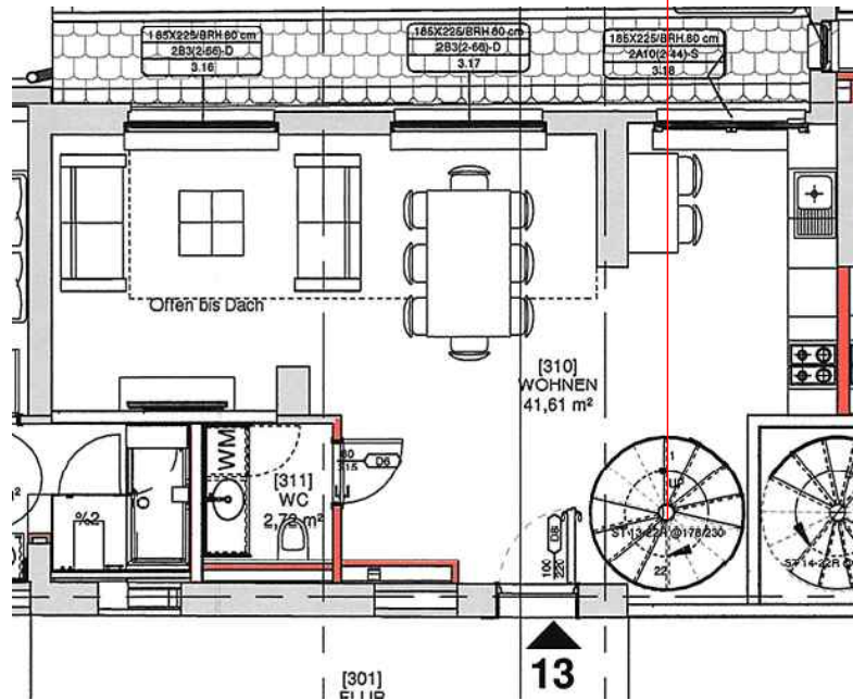
Wohnung 13, Grundriss 3.OG
