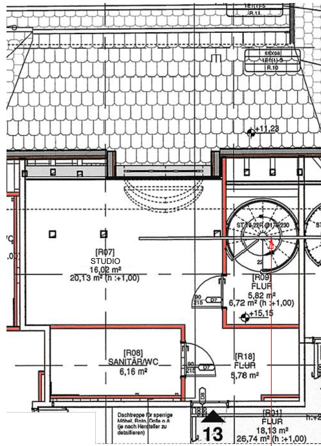
Wohnung 13, Grundriss DG
