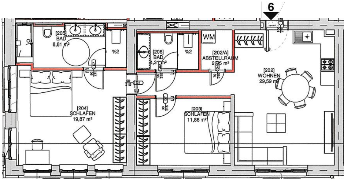
Wohnung 6, Grundriss 2.OG
