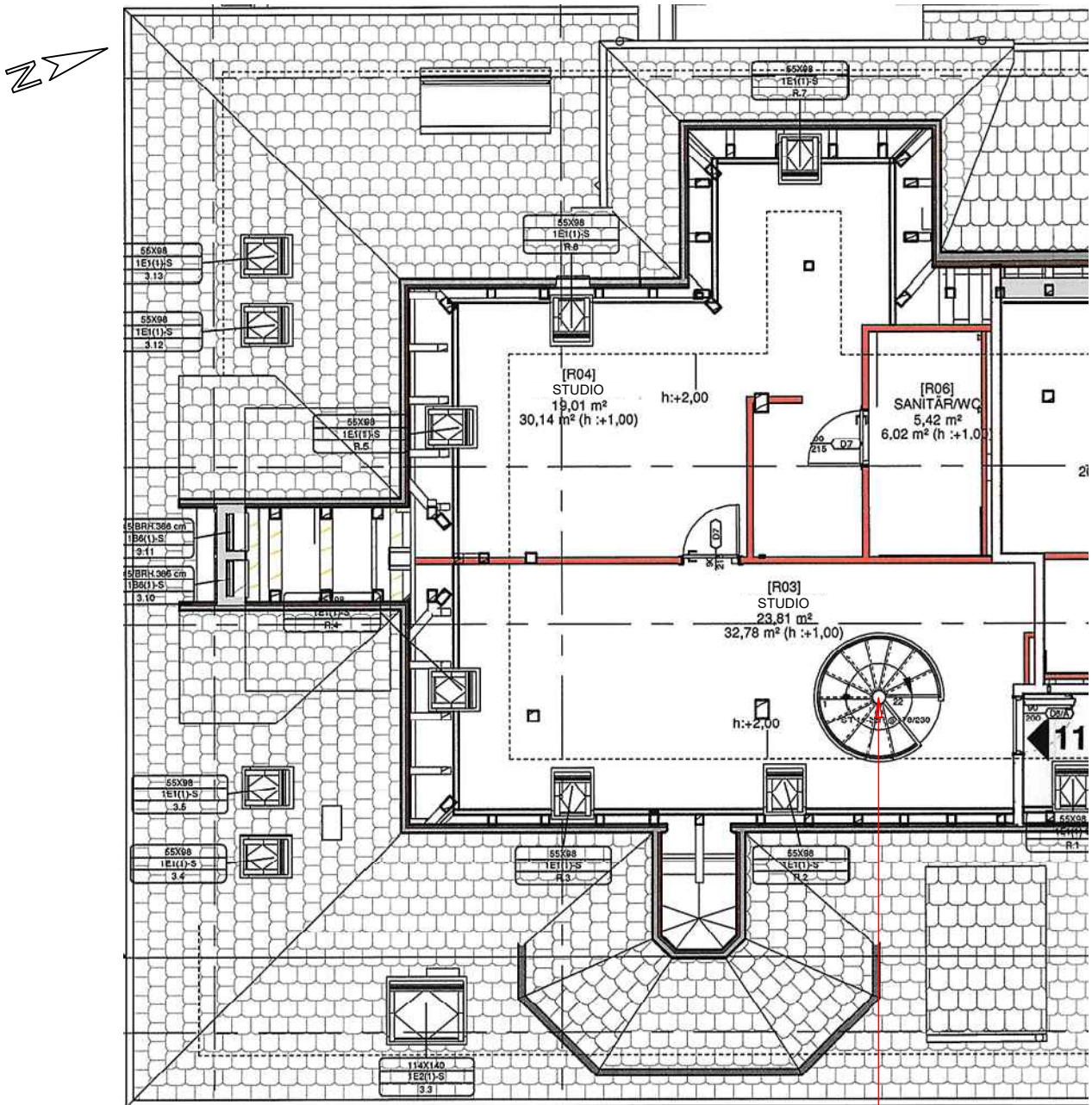
▲ Wohnung 11, Grundriss DG
