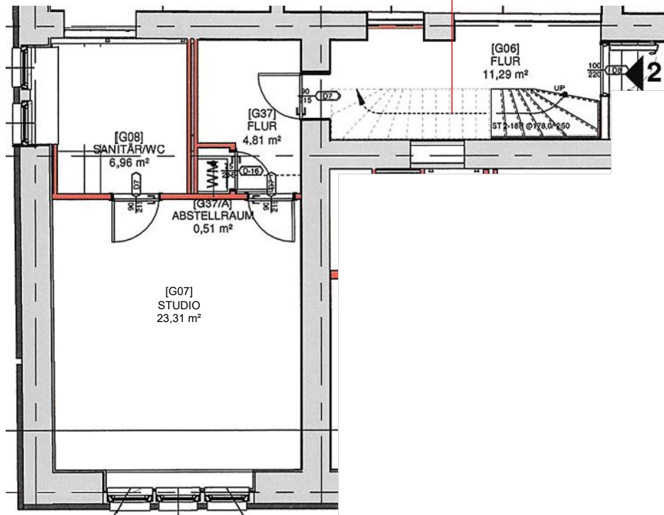
Wohnung 2, Grundriss EG
