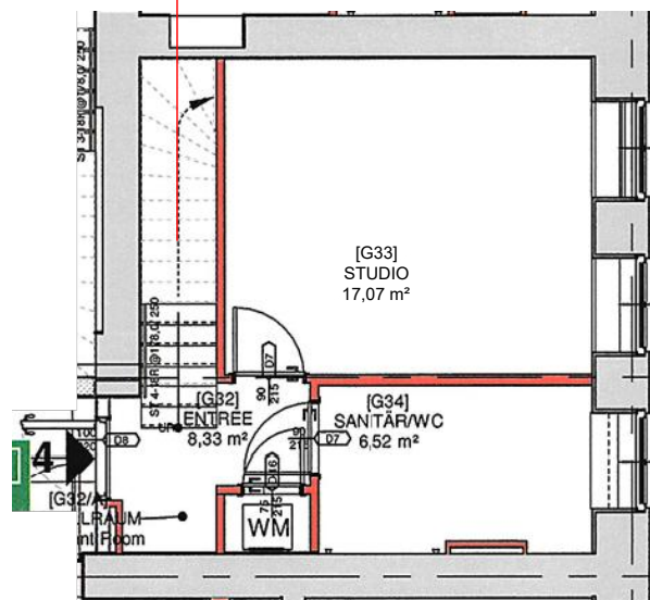
Wohnung 4, Grundriss EG
