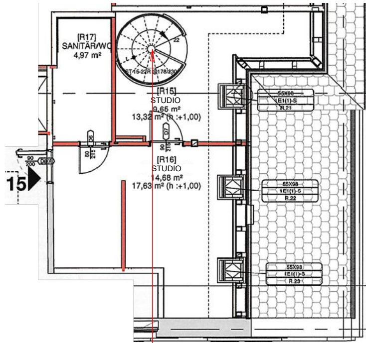
Wohnung 15, Grundriss DG
