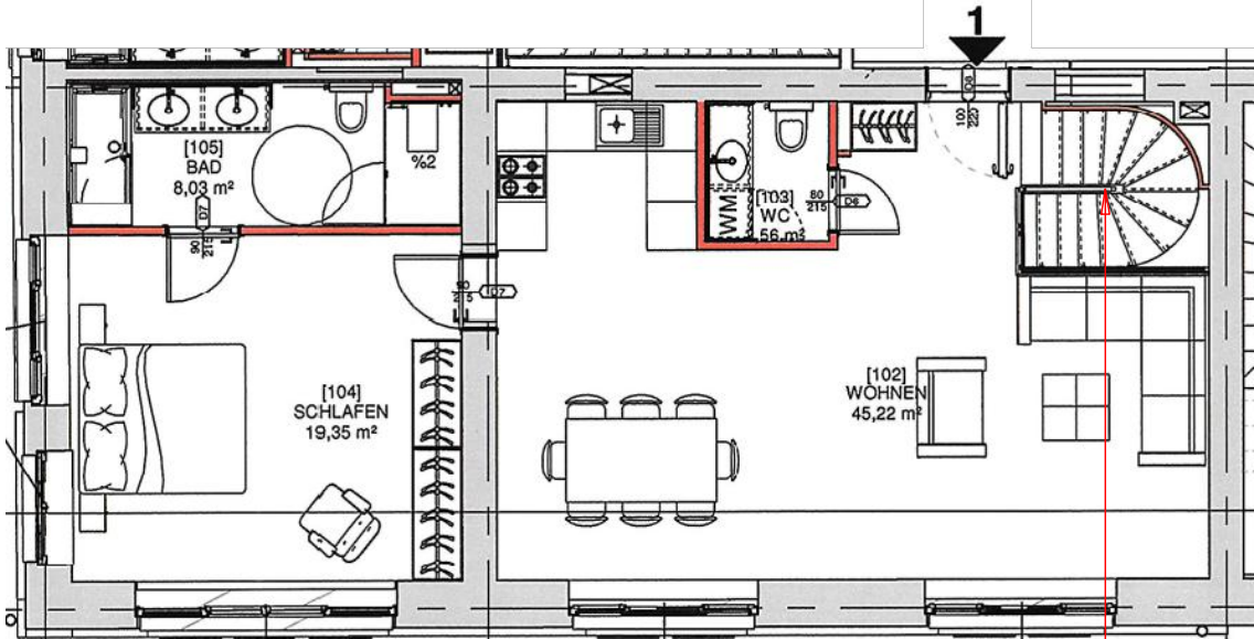
Wohnung 1, Grundriss 1.OG
