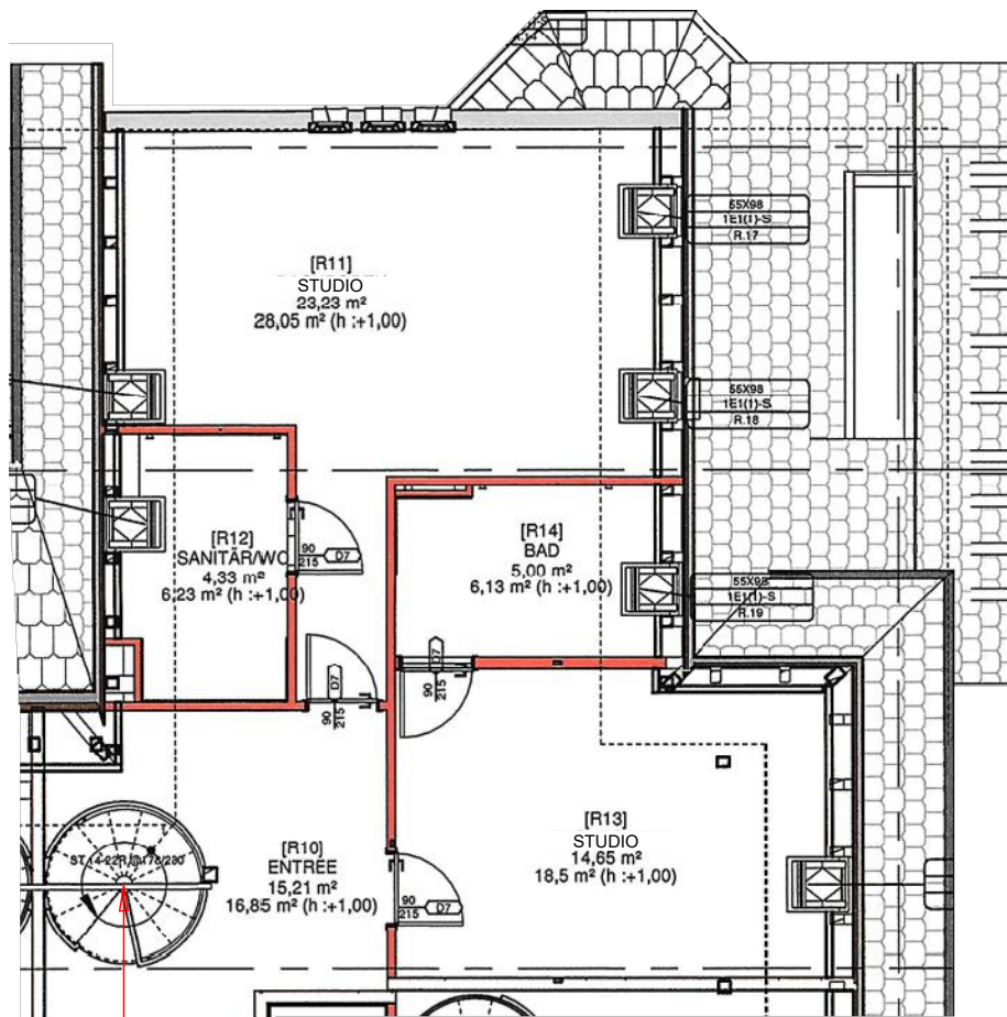
Wohnung 14, Grundriss DG
