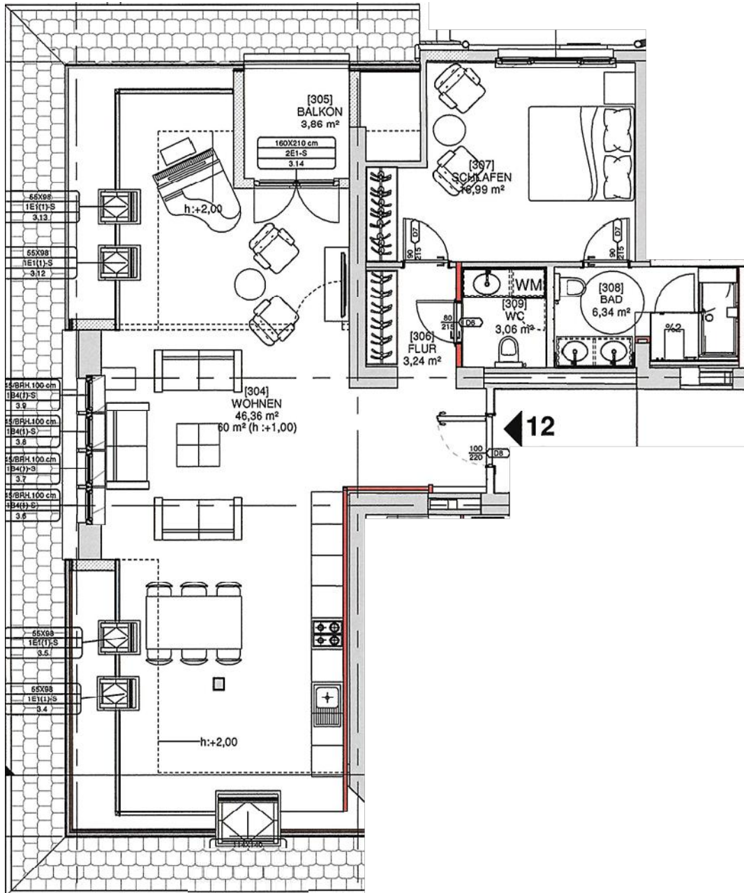
Wohnung 12, Grundriss 3.OG
