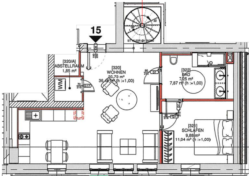
Wohnung 15, Grundriss 3.OG
