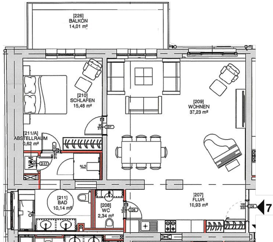
Wohnung 7, Grundriss 2.OG
