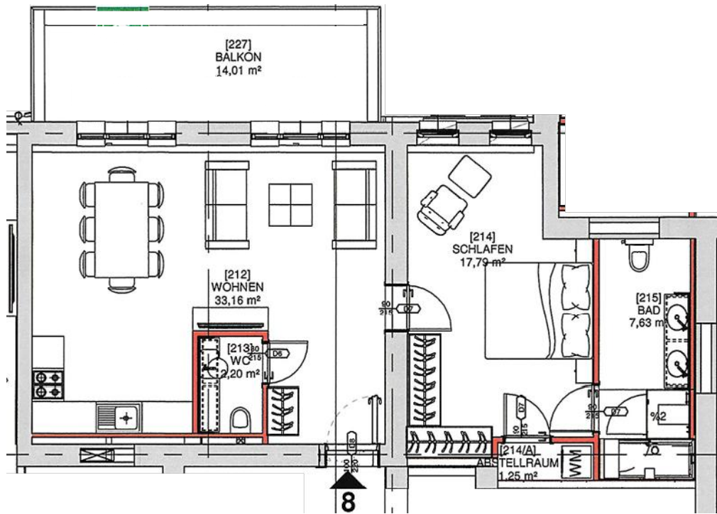
Wohnung 8, Grundriss 2.OG
