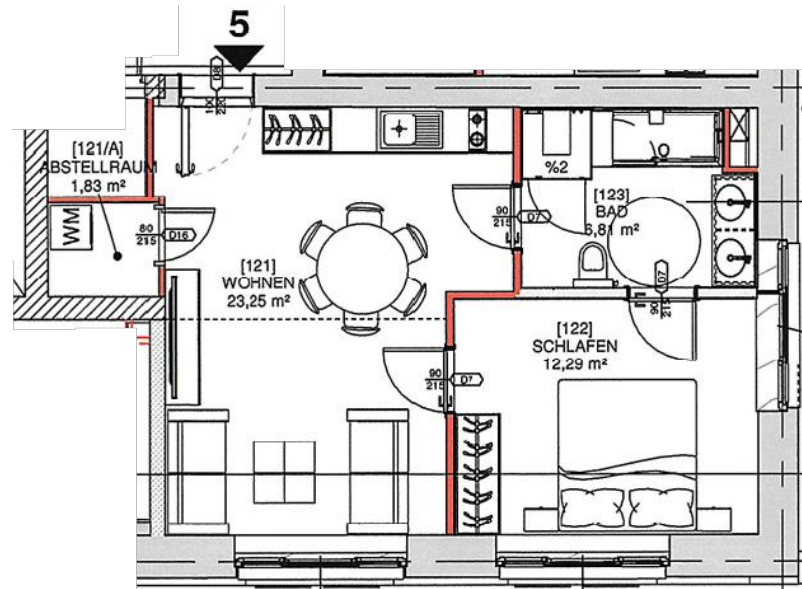
Wohnung 5, Grundriss 1.OG
