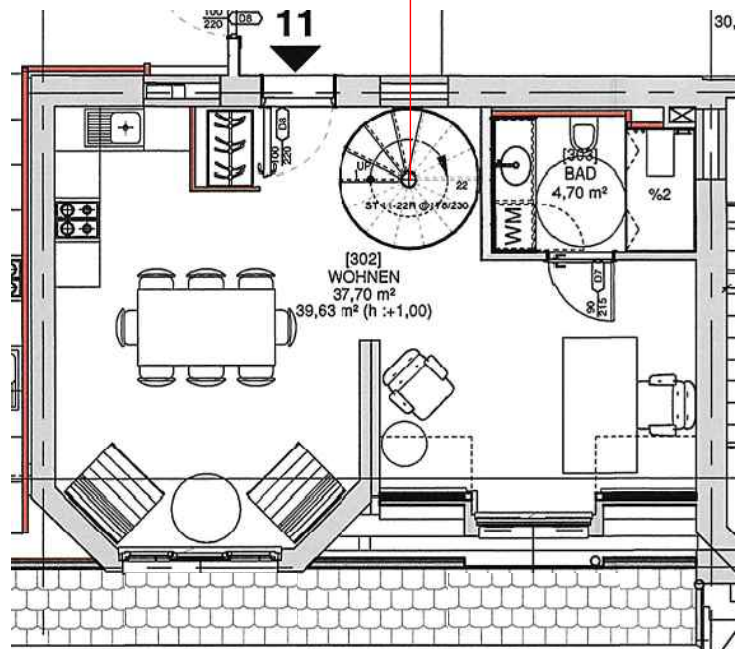
Wohnung 11, Grundriss 3.OG ▶
